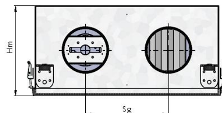
Вид слева
