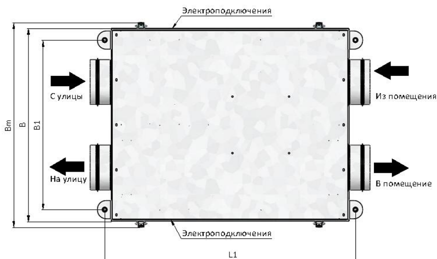
Вид сверху
