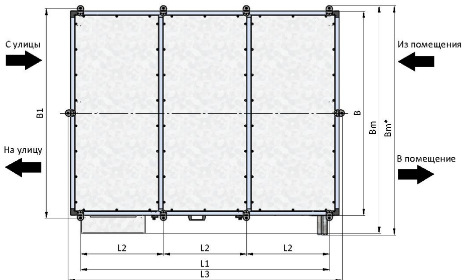
Вид сверху
