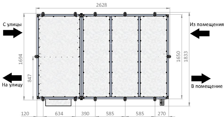
Вид сверху
