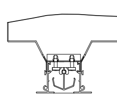
Крепление с траверсой (Z)
