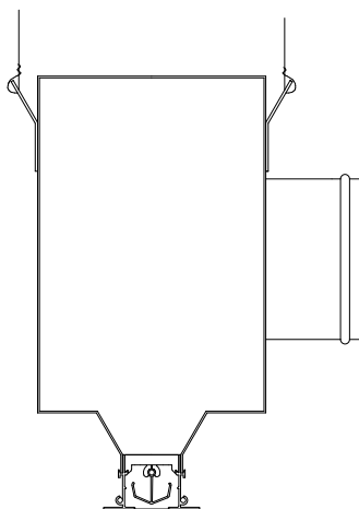
Монтаж присоединительной камеры с помощью подвесов (P)
